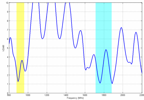
VSWR
